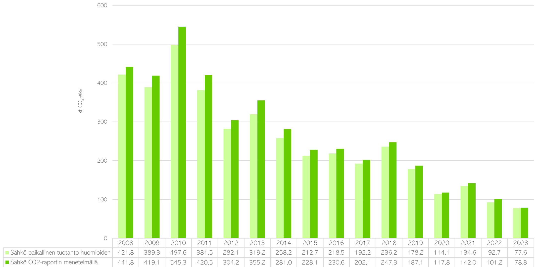
Kuva 9. Rauman sähkönkulutuksen päästöt vuosina 2008–2023 (sisältäen kuluttajien sähkönkulutuksen, teollisuuden sähkönkulutuksen, sähkölämmityksen ja maalämpöpumppujen sähkönkäytön) laskettuna CO2-raportin menetelmällä ja paikallinen tuotanto huomioiden (eli oletetaan, että Raumalla tuotettu sähkö on kulutettu Raumalla). (CO2-raportti, 2025)
