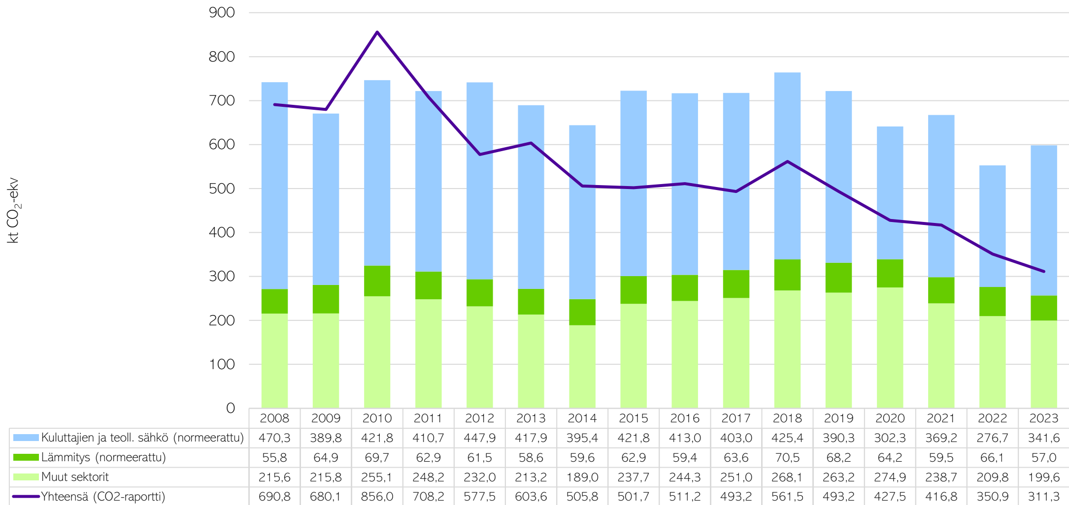
Kuva 5. Rauman päästöt normeerattuna käyttäen lämmitystarpeelle ilmastollista vertailukautta (1981–2010) ja sähkönkulutukselle keskimääräistä päästökerrointa (pylväät). Sähkölämmitys ja maalämpö ovat mukana lämmityksessä, sähkö sisältää kuluttajien ja teollisuuden sähkönkulutuksen. "Muut sektorit" sisältää sektorit, joihin normeeraus ei vaikuta (liikenne, teollisuus ja työkoneet, maatalous, jätehuolto). Viivalla on esitetty normeeraamattomat päästöt yhteensä. (CO 2 -raportti, 2025).
