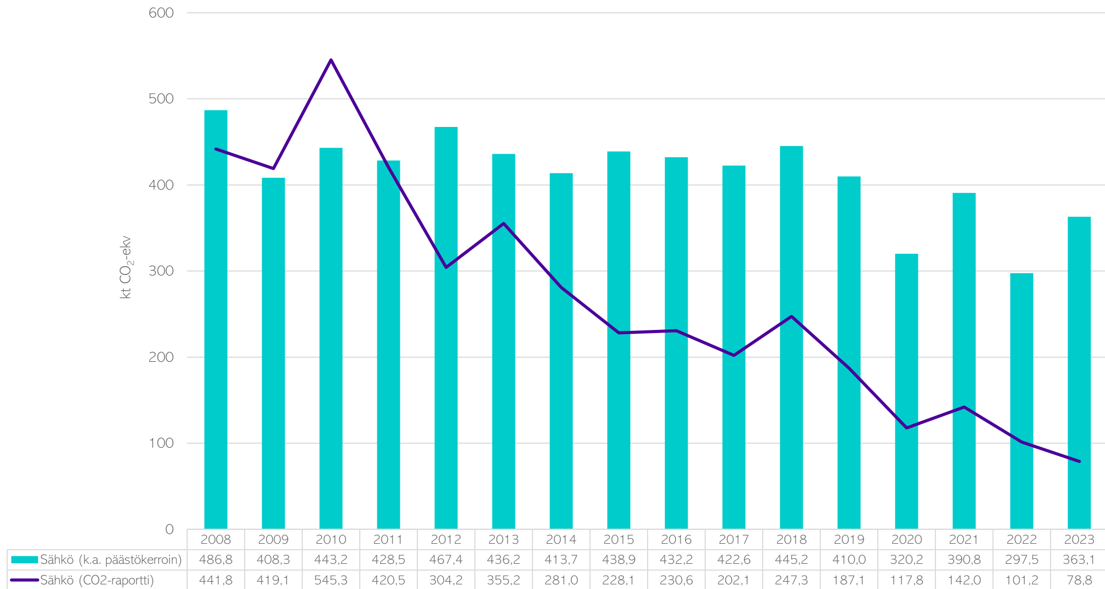
Kuva 7. Rauman sähkönkulutuksen päästöt vuosina 2008–2023 (sisältäen kuluttajien sähkönkulutuksen, teollisuuden sähkönkulutuksen, sähkölämmityksen ja maalämpöpumppujen sähkönkäytön) laskettuna CO2-raportin menetelmällä (viiva) ja keskimääräistä päästökerrointa käyttäen (pylväät). (CO2-raportti, 2025).
