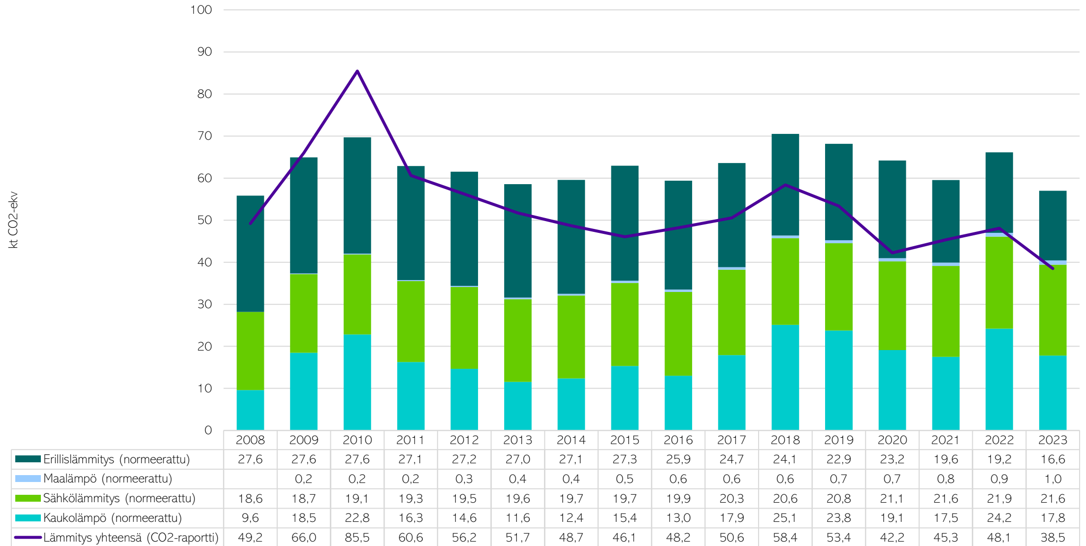
Kuva 11. Lämmityksen päästöt vuosina 2008–2023 korjattuna vastaamaan ilmastollista vertailukautta 1981–2010 ja käyttäen sähkölämmitykselle ja maalämmölle keskimääräistä päästökerrointa. Normeeraamattomat lämmityksen päästöt yhteensä on esitetty viivalla. (CO 2 -raportti, 2025).
