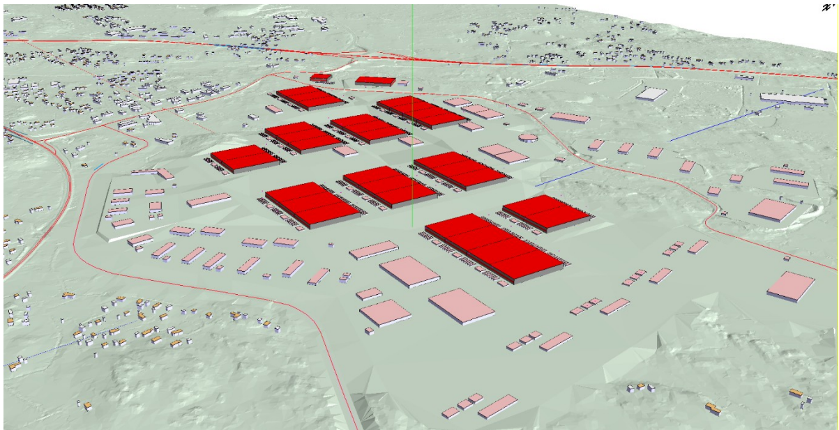
Kuva 2. Näkymä melun laskentamallin maastomalliin kaakon suunnasta. Konesalit esitetty tummemmalla punaisella.
